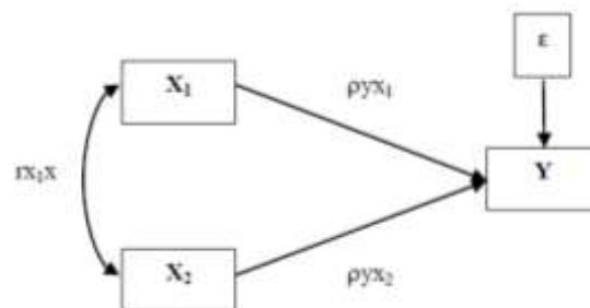
Gambar 1 Analisis Jalur
