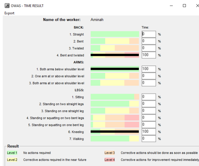
Gambar 3. Output rekomendasi tindakan dari metode OWAS
