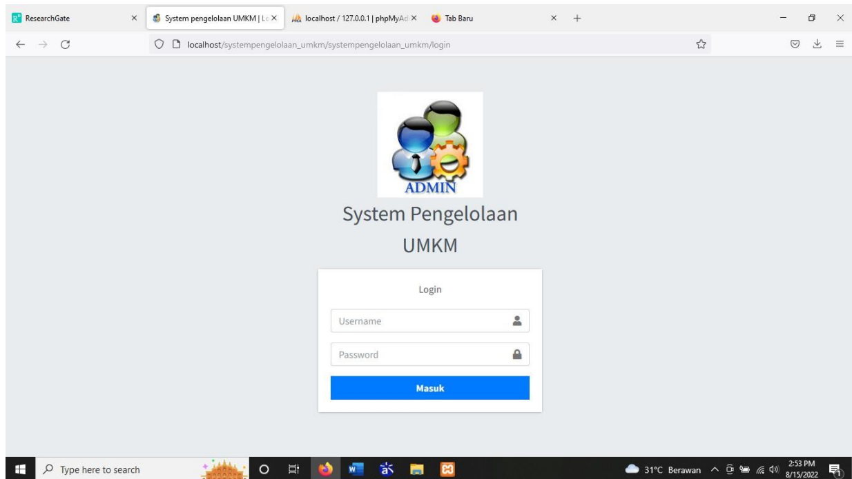
Gambar 4.3 Tampilan depan
