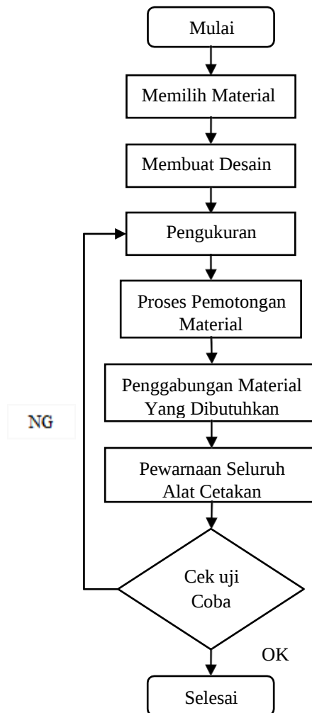
FlowChart Pembuatan tong sampah bakar 2)
