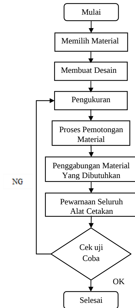
Gambar 3 FlowChart Pembuatan tong sampah bakar
