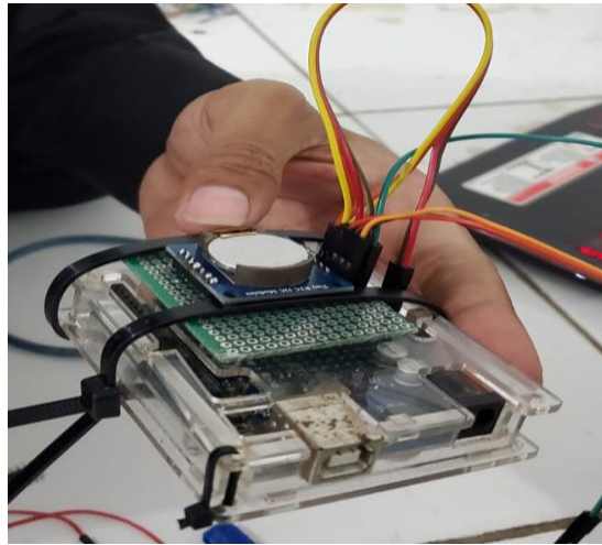
Gambar 2.2 Perakitan Komponen
